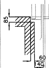
DETAL Y Drzwi 0,2,3,4
